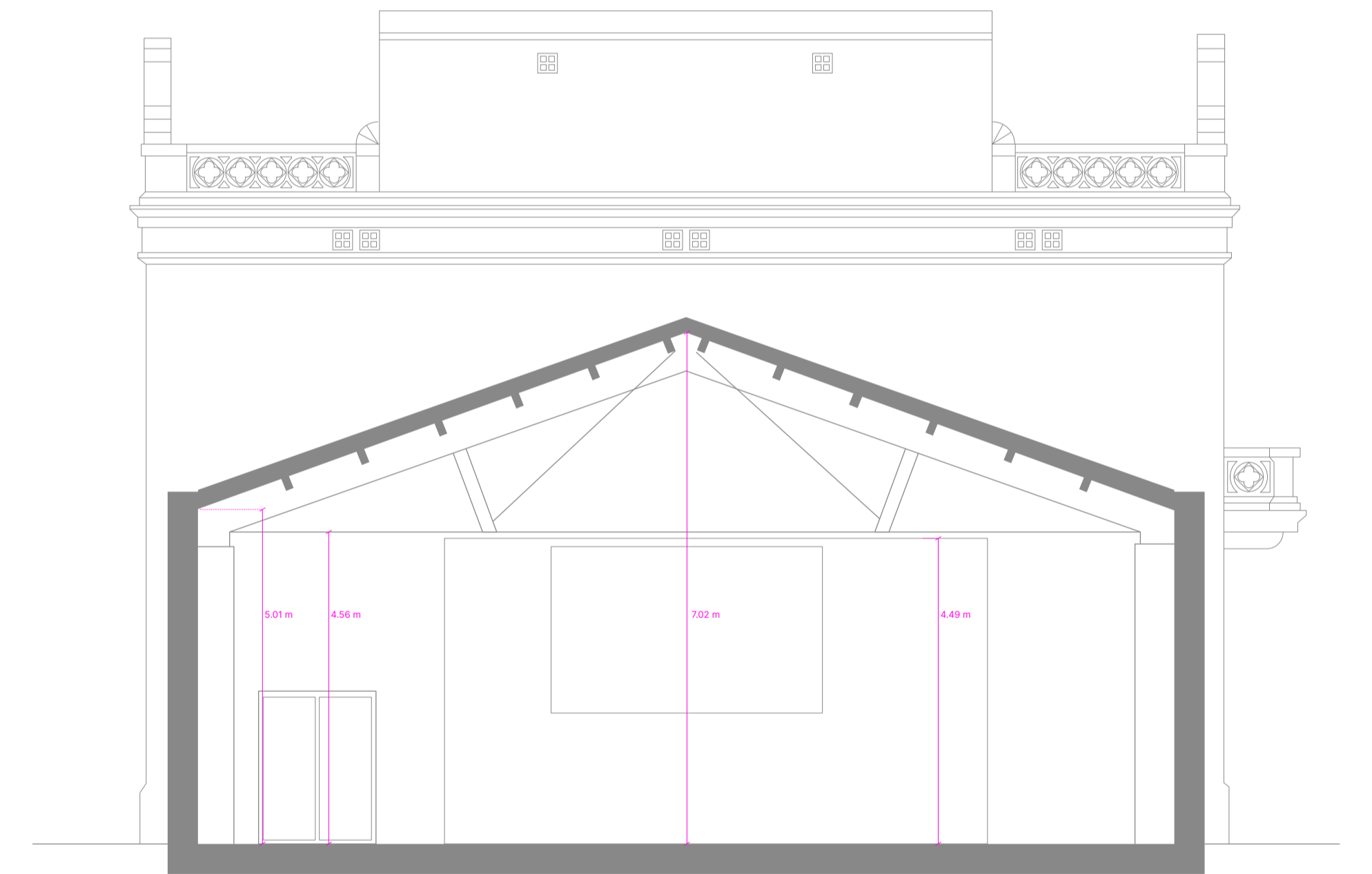
SECCIÓN TRANSVERSAL - EL TALLER
