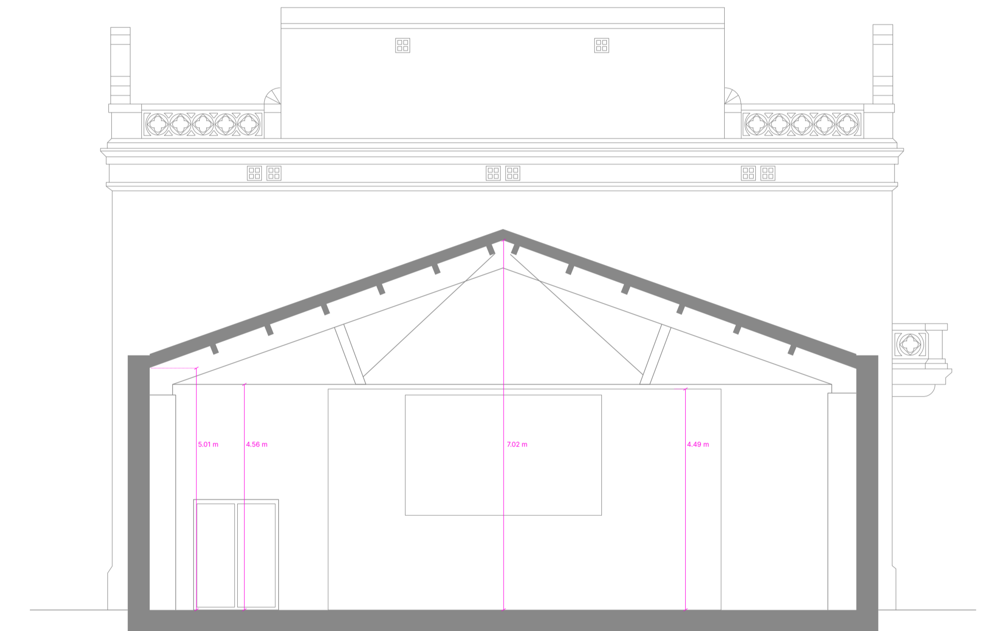
SECCIÓ TRANSVERSAL - EL TALLER
