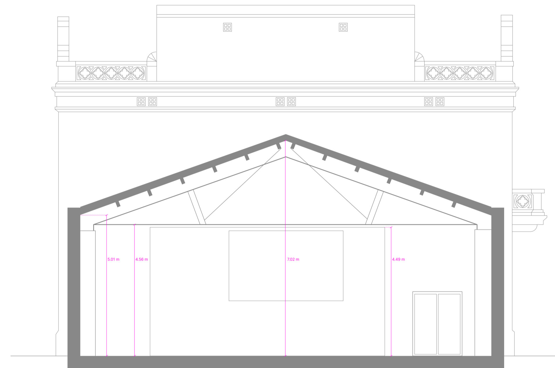
SECCIÓ TRANSVERSAL - LA FUSTERIA
